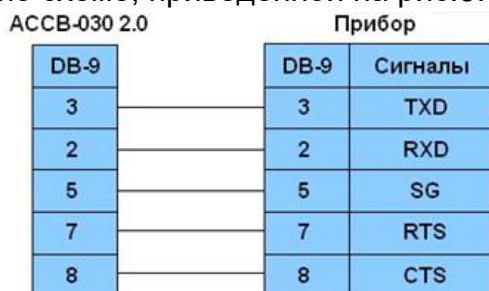
Рис.9. Подключение прибора по интерфейсу RS-232.
