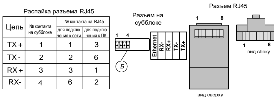
Рис.А.4. Обозначения коммутационных элементов на субблоке вычислителя адаптера ИВК-СК
