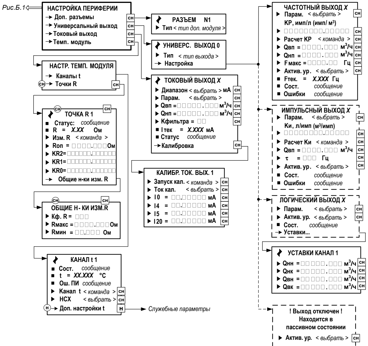
Рис.Б.5. Меню «Настройка периферии».
