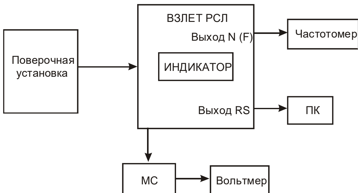
Рис.3. Схема соединений при поверке расходомера.
