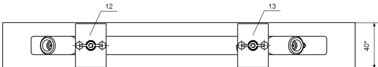
г) вид сверху линейки 150 мм
