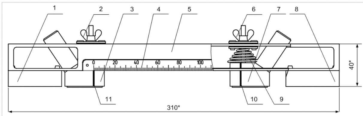
б) вид сбоку линейки 150 мм
