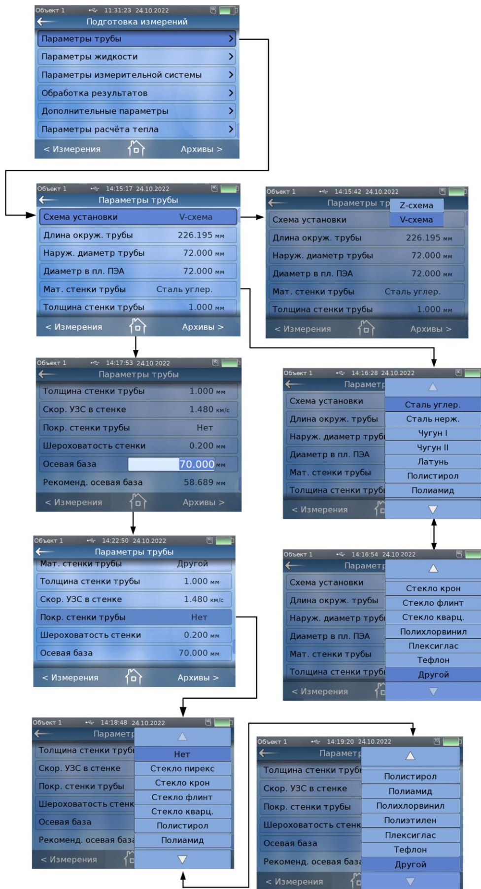
Рис.Г.2. Меню «Подготовка измерений» / «Параметры трубы»
